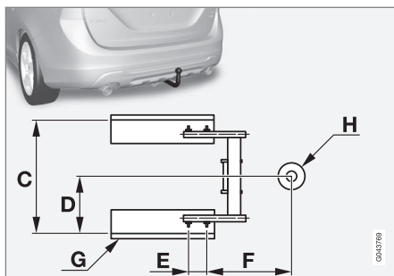
Medidas, pontos de fixação (mm)
