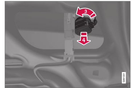
Lampengehäuse rechts.
