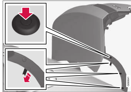
Der Kunststoffschutz des Scharniers ist mit einem Kunststoffniet und drei Schnappverschlüssen befestigt.
