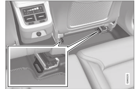
Lage der Befestigungspunkte für den Rücksitz.
