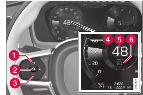
Tasten und Symbole der Funktion 27 .
