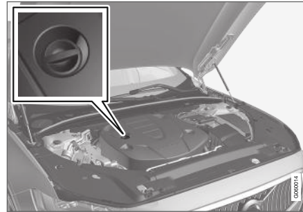
Einfüllrohr 12 .
