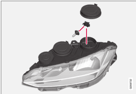
Linker Scheinwerfer.
