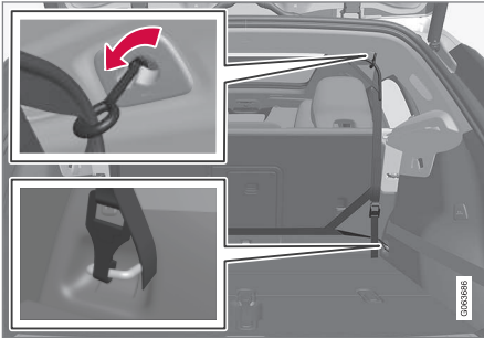
Hátso rögzítés.
