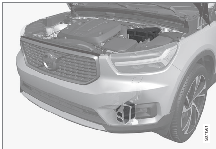
A 12 voltos segédakkumulátor lent a motorterében található. Az indítóakkumulátor itt látható (fent).
