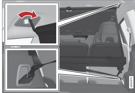
뒤쪽 고정.
