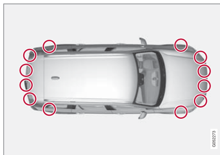
駐車感知器位置 140。
