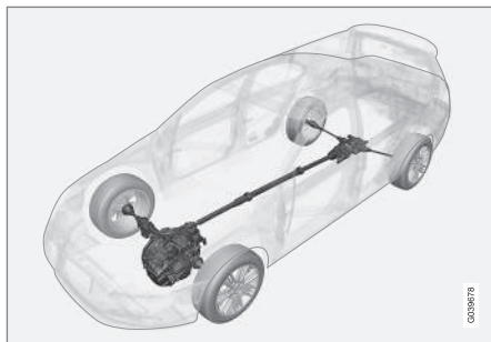
Principio AWD 7 .
