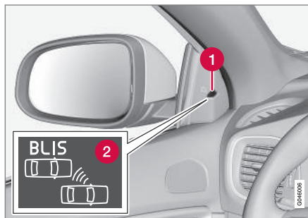
Ubicación de la luz BLIS 22 .
