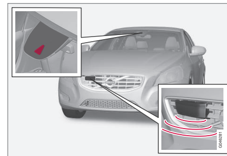
Sensor de cámara y de radar 20 .
