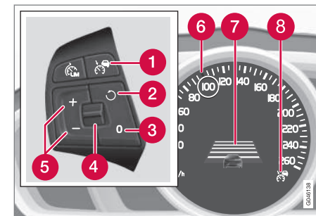
Adaptiv farthållare med Fartbegränsare 9 .
