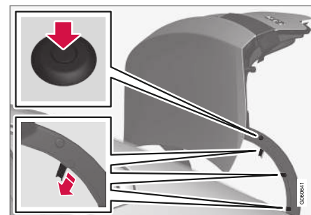
La protección de plástico de la bisagra va montada con un remache plástico y tres cierres de resorte.
