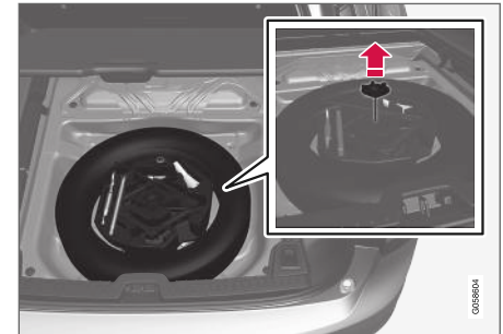
Imagen esquemática: La forma del bloque de gomaespuma puede variar en función del modelo de vehículo.
