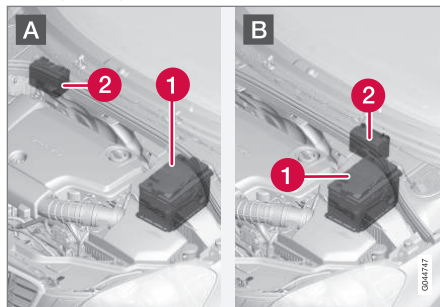
A: Vasemmalta ohjattava auto. B: Oikealta ohjattava auto. (1) Käynnistysakku 17 (2) Apuakku.
