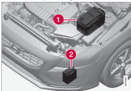
(1) Startbatteri 15 (2) Stödbatteri
