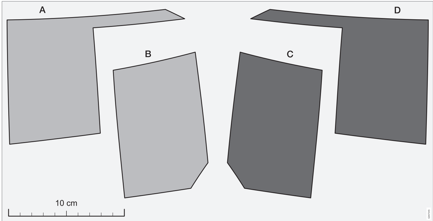
Mallar för halogenstrålkastare
