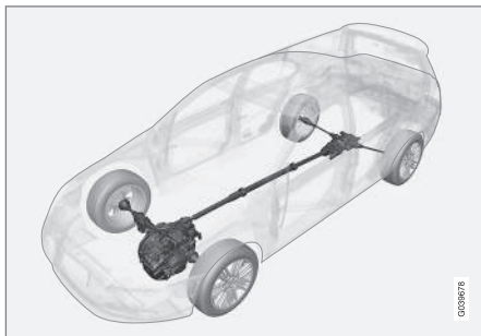
AWD-princip 9 .
