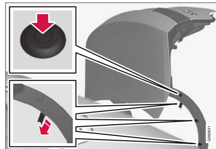
Plastový kryt závěsu je připevněn pomocí plastového nýtu a tří západek.
