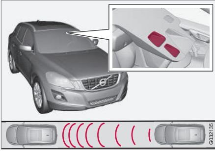
Lazer sensörü verici ve alıcı penceresi 12 .
