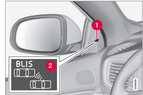
Positie BLIS-lampje 21 .
