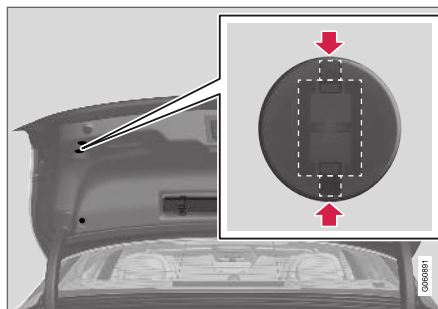
A parte retangular dos cliques está orientada na direção do comprimento do automóvel.
