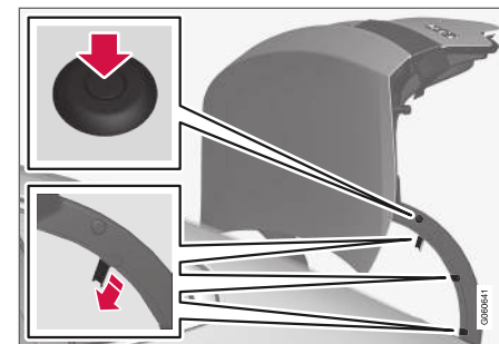
O resguardo de plástico da dobradiça é montado com um rebite de plástico e três trincos.
