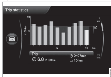
Статистика поездок 28
