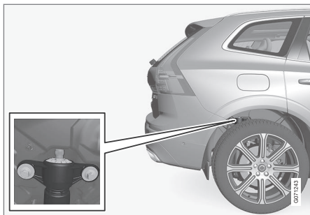
어저스터 노브의 위치, 뒤쪽 휠
