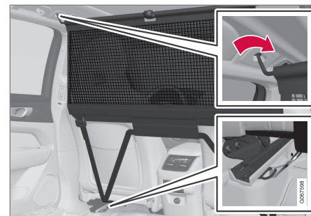
전방에 장착하기.
