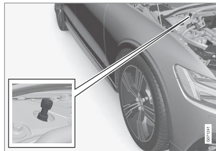
어저스터 노브의 위치, 앞쪽 휠
