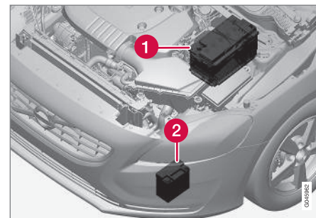
(1) Batería de arranque 17 (2) Batería de apoyo
