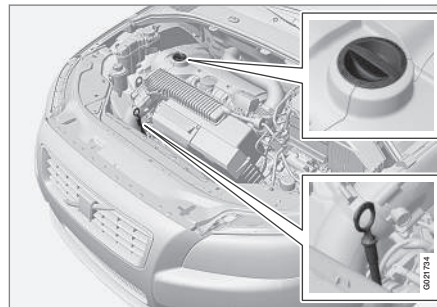
Måttsticka och påfyllningsrör.
