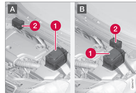
A: Vänsterstyrd bil. B: Högerstyrd bil. (1) Startbatteri 17 (2) Stödbatteri.
