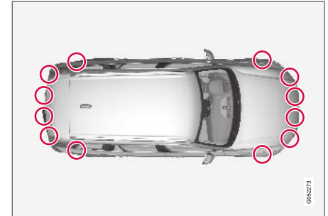
Pysäköintitunnistimien sijainti 125 .
