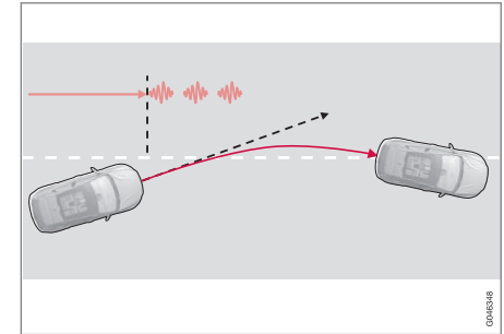
La funzione LKA sterza e avverte il conducente mediante pulsazioni al volante 24 .
